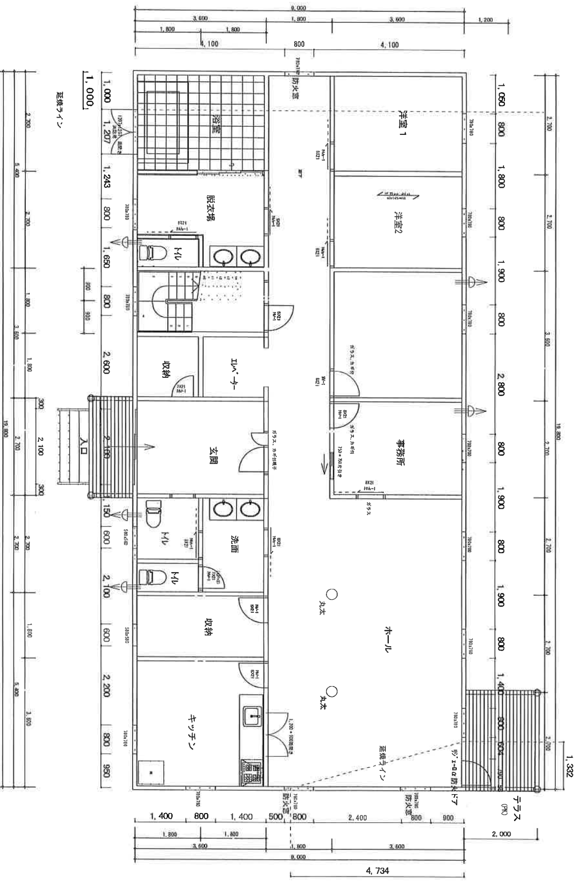
1階平面図 1/100 178.2㎡
